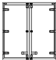
Familia OT2 (dos batientes)
